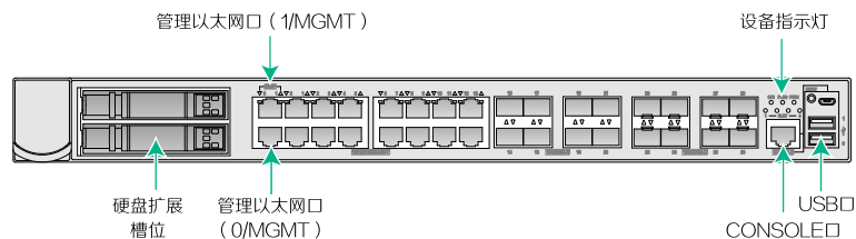
F5000-G15设备外观图
